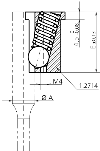
INSERT DIMENSIONS
